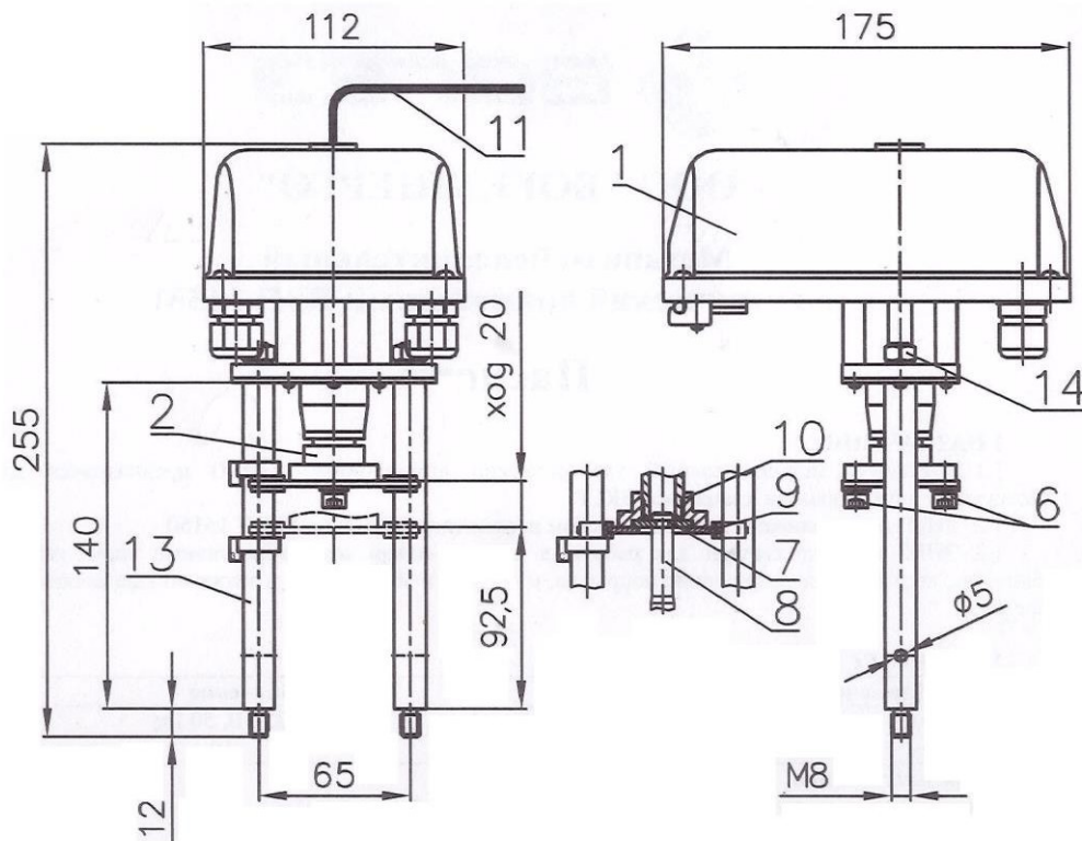
Рисунок 1 – МИЭП-1-1600
