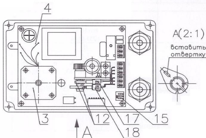
Рисунок 1 – МИЭП-1-1600
